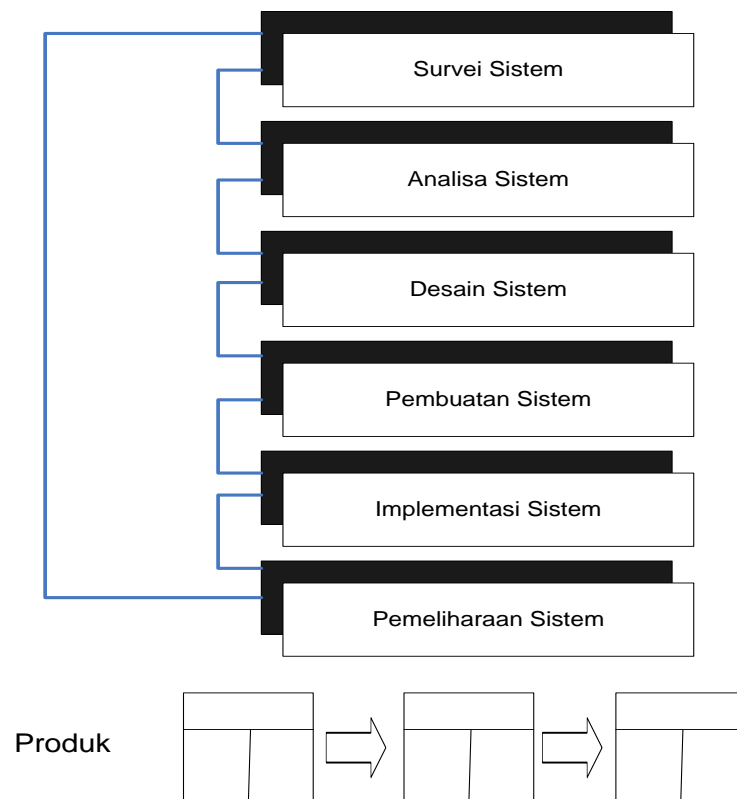
Gambar 1.4 Iterasi (2004: 63)
